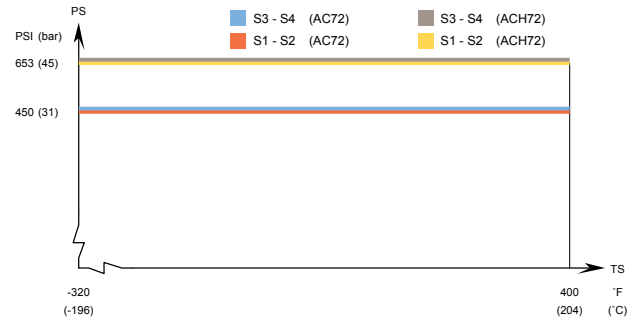
AC72/ACH72 – UL 인증 압력/온도 그래프
