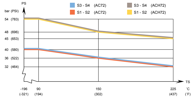
AC72/ACH72 – PED 인증 압력/온도 그래프 /
