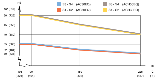
AC30EQ/ACH30EQ – PED 인증 압력/온도 그래프
