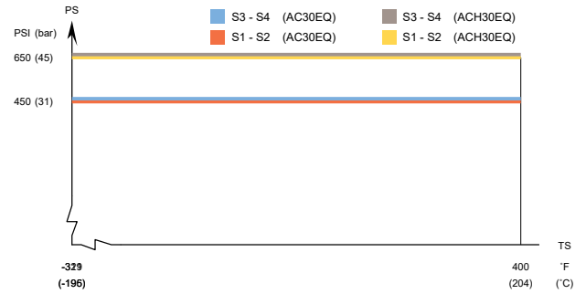
AC30EQ/ACH30EQ – UL 인증 압력/온도 그래프
